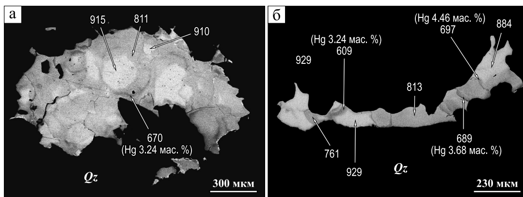
Рис. 4. Пробность (‰) и содержание Hg (мас. %) в зернах золота из золотосульфидно-кварцевых жил месторождения Кызык-Чадр. Снимки в режиме BSE.
