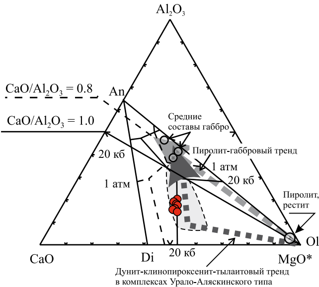
Рис. 2. Положение фигуративных точек составов израндитов в координатах CaO–Al 2 O 3 –MgO*.
