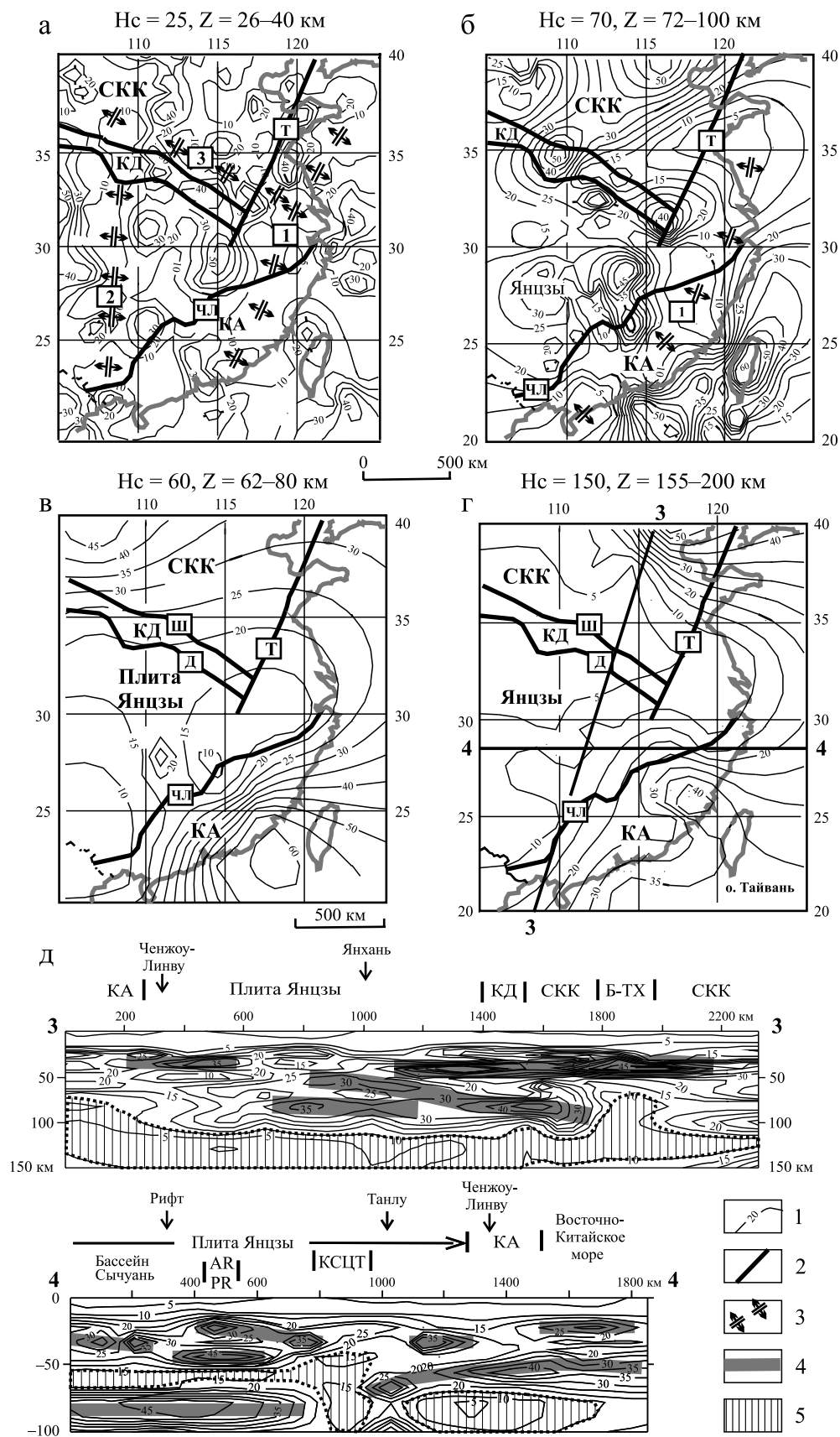
Рис. 6. Плотностная контрастность тектоносферы на юго-востоке Азиатского континента: карты-срезы (а-г) и разрезы (д) 3D модели плотностной контрастности.
