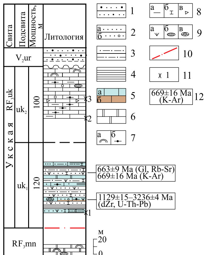
Рис. 3. Литолого-стратиграфическая колонка отложений укской свиты в правобережье р. Басу и ее притока р. Манайсу в 600 м восточнее хут. Кулмас вдоль автотрассы Уфа–Инзер–Белорецк. Обн. 1–3.
