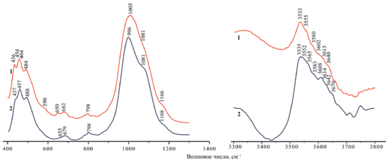
Рис. 8. ИК-спектры глауконита.
